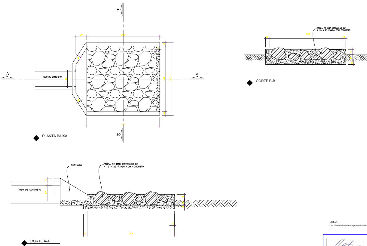
DETALHE - DISSIPADOR DE ENERGIA
