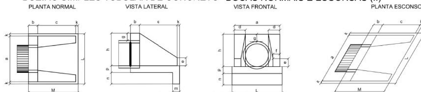
DIMENSÕES E CONSUMOS MÉDIOS PARA UMA UNIDADE
