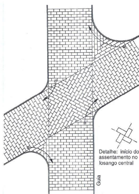
Figura 02 – Cruzamentos Esconsos
