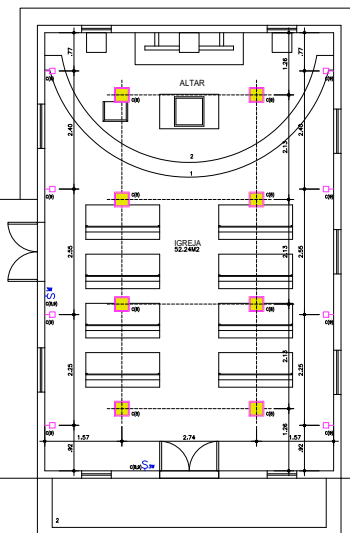
PLANTA LUMINOTÉCNICA IGREJA ESCALA 1/50
