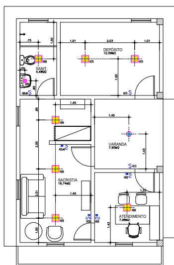
PLANTA LUMINOTÉCNICA SACRISTIA ESCALA 1/50
